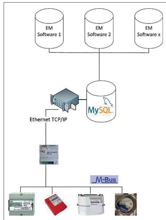
Abb.: Grundkonzept der Zählerstruktur mit Datenbank und Visualisierung
